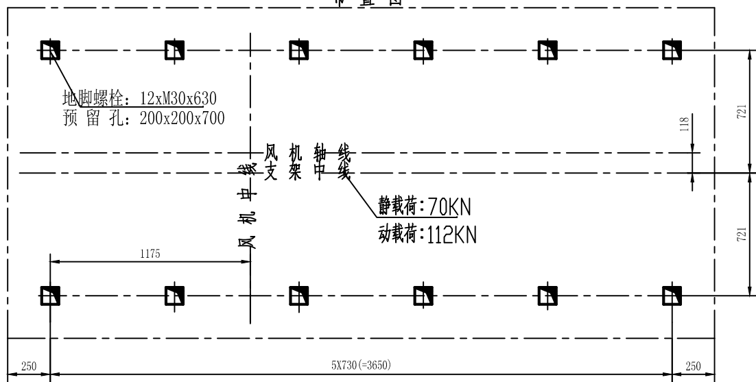
基础平面 布置图
